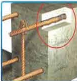
Chemical Anchor Rebar ချိတ်ဆက်နည်းလမ်း
